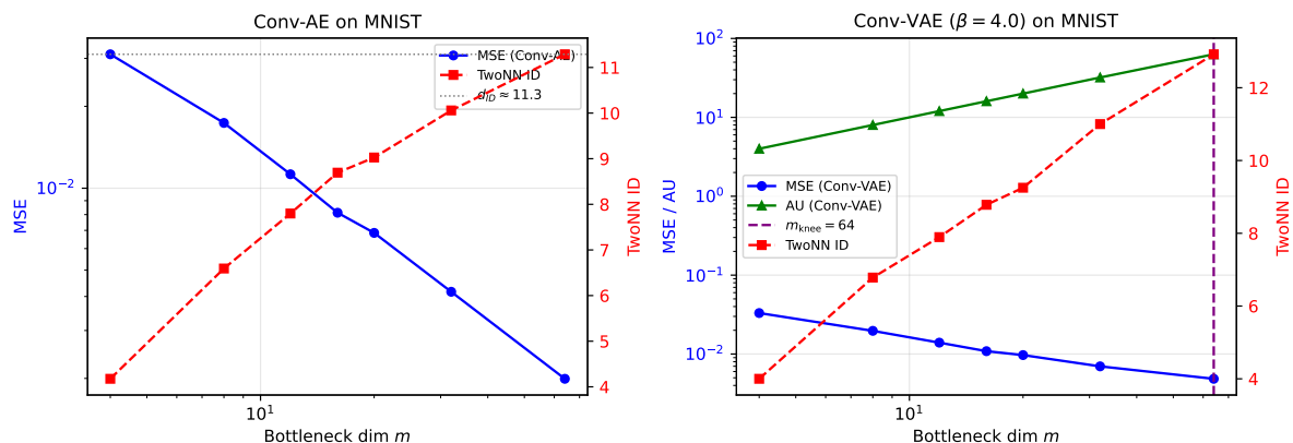
図 10: Exp-Conv-AE: Conv-AE (左) \cdot Conv-VAE (右) における MSE, AU, TwoNN ID の m 依存性 (MNIST, 100 エポック). Conv-AE では \text{AU} = m (全次元活性) が確認され, TwoNN ID が m \geq 32 で \approx 11 に収束する. Conv-VAE では \text{AU} \approx m (100 エポックの収束不足により飽和なし).
