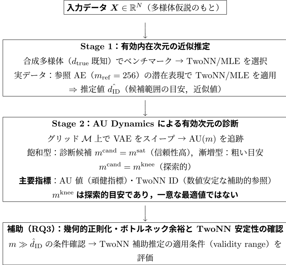
図 1: 有効潜在次元の診断パイプライン. 診断候補次元 m^{\text{cand}} はボトルネック次元の一意な最適解ではなく, 多指標 (AU 値 \cdot TwoNN ID \cdot m^{\text{knee}} ) を総合した診断上の候補である.
