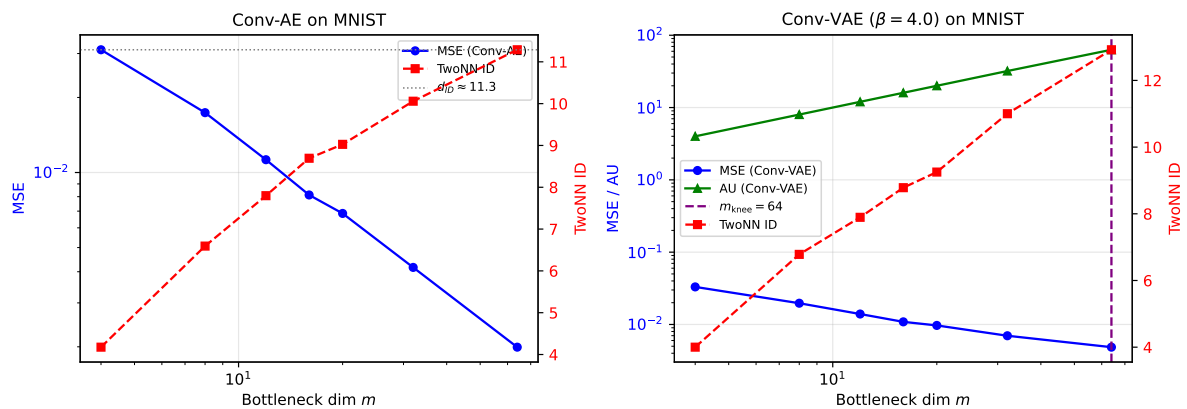
図 10: Exp-Conv-AE: Conv-AE (左) \cdot Conv-VAE (右) における MSE, AU, TwoNN ID の m 依存性 (MNIST, 100 エポック). Conv-AE では AU = m (全次元活性) が確認され, TwoNN ID が m \geq 32 で \approx 11 に収束する. Conv-VAE では AU \approx m (100 エポックの収束不足により飽和なし).
