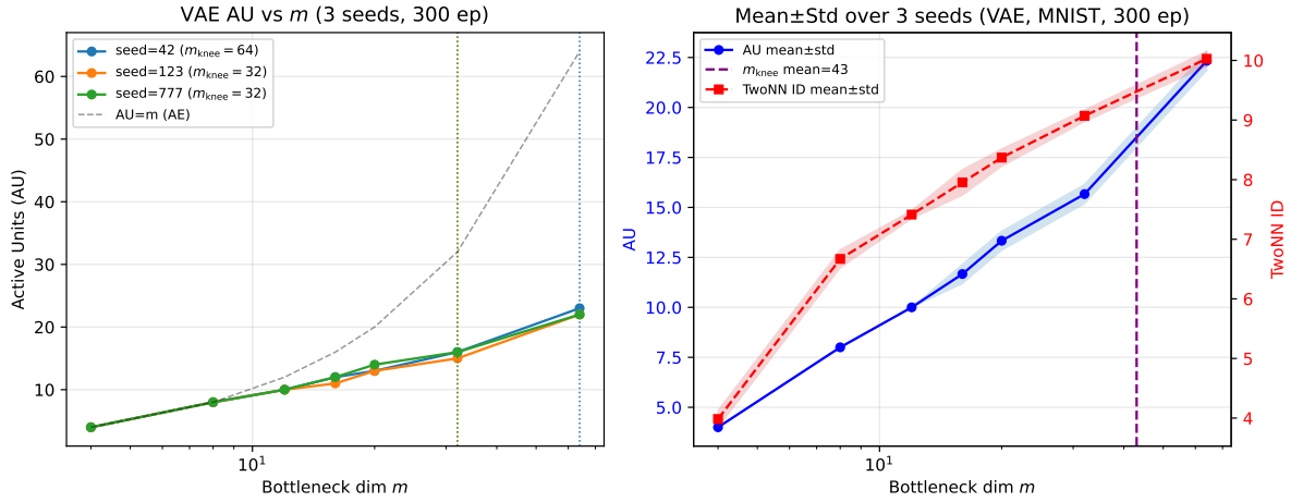
図 4: E4-300ep-multiseed : MNIST VAE の AU パターン (3 シード, 300 エポック). 左: 各シードの AU vs m (点線は m^{\text{knee}} ); 右: 平均 \pm 標準偏差バンド. AU・TwoNN ID のバンドは非常に狭いが, m^{\text{knee}} はシード間で 32~64 に変動する.
