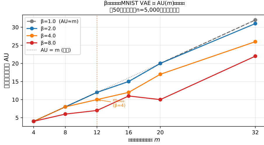
図 11: \beta 感度分析：MNIST VAE の AU vs m ( \beta \in \{1, 2, 4, 8\} , 50 エポック, サブセット). \beta = 1 では AU \approx m (正則化不足), \beta = 4 では m_{\text{knee}} = 12 (垂直破線), \beta = 8 では m < 8 で AU が過度に抑制される兆候が見られる.
