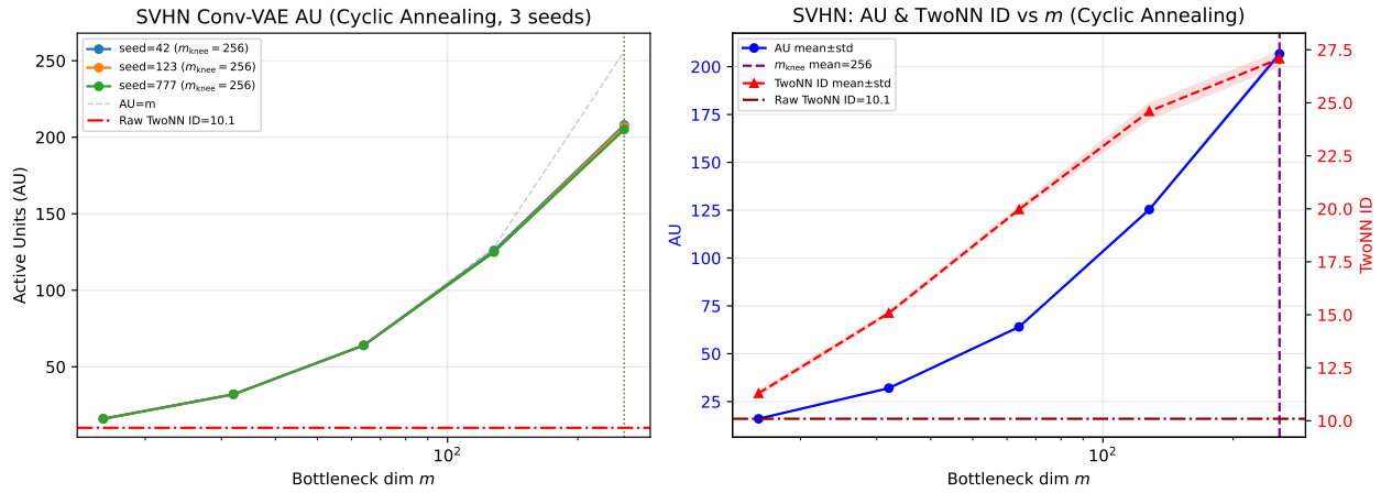
図 10: EJ : SVHN Conv-VAE (KL サイクリックアニーリング) における AU・TwoNN ID の m 依存性 (3 シード).
