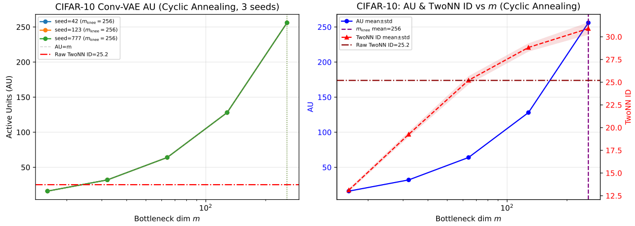
図 9: EI : CIFAR-10 Conv-VAE (KL サイクリックアニーリング) における AU・TwoNN ID の m 依存性 (3 シード). TwoNN ID は Pope ら [17] の報告値 ( d_{\text{ID}} \approx 26 ) と収束傾向を示す.
