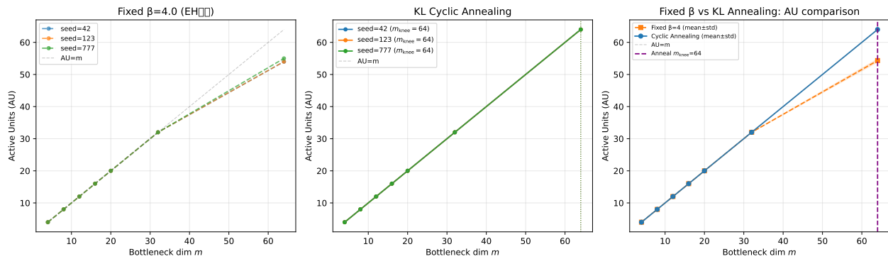
図 8: EK：固定 \beta （左）vs KL サイクリックアニーリング（中央）の各シード AU 曲線，および平均比較（右）．固定 \beta では m = 64 のみで部分的崩壊（ AU \approx 54 ）が生じるが，アニーリングでは全次元が常に活性（ AU = m ）となり， m \in [4, 64] の範囲ではいずれの条件でも明確な AU 飽和（AU が m を下回るプラトー）は観測されなかった．
