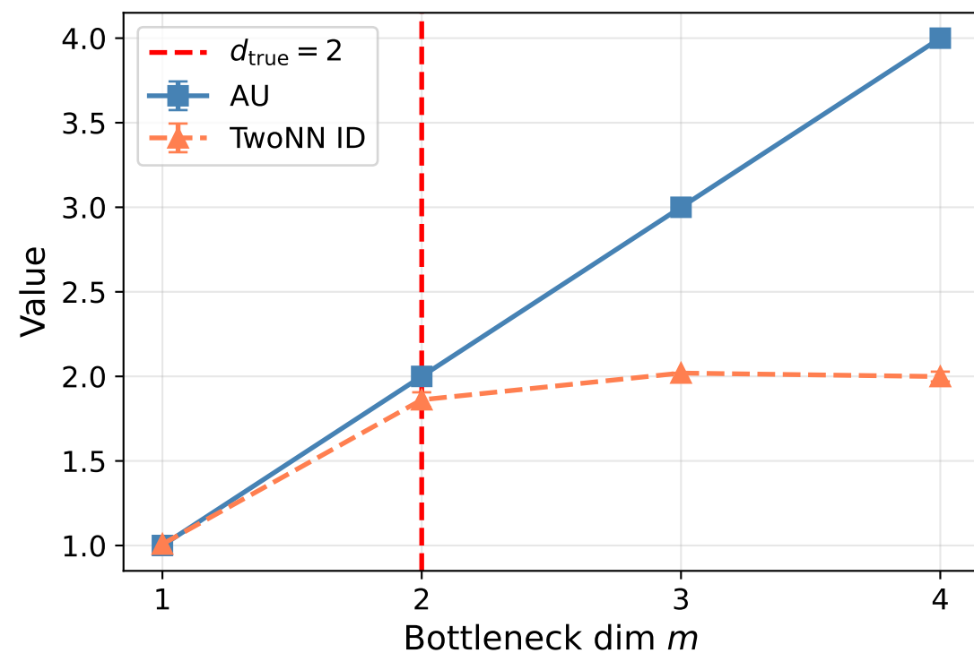
Torus: AU & ID vs m
