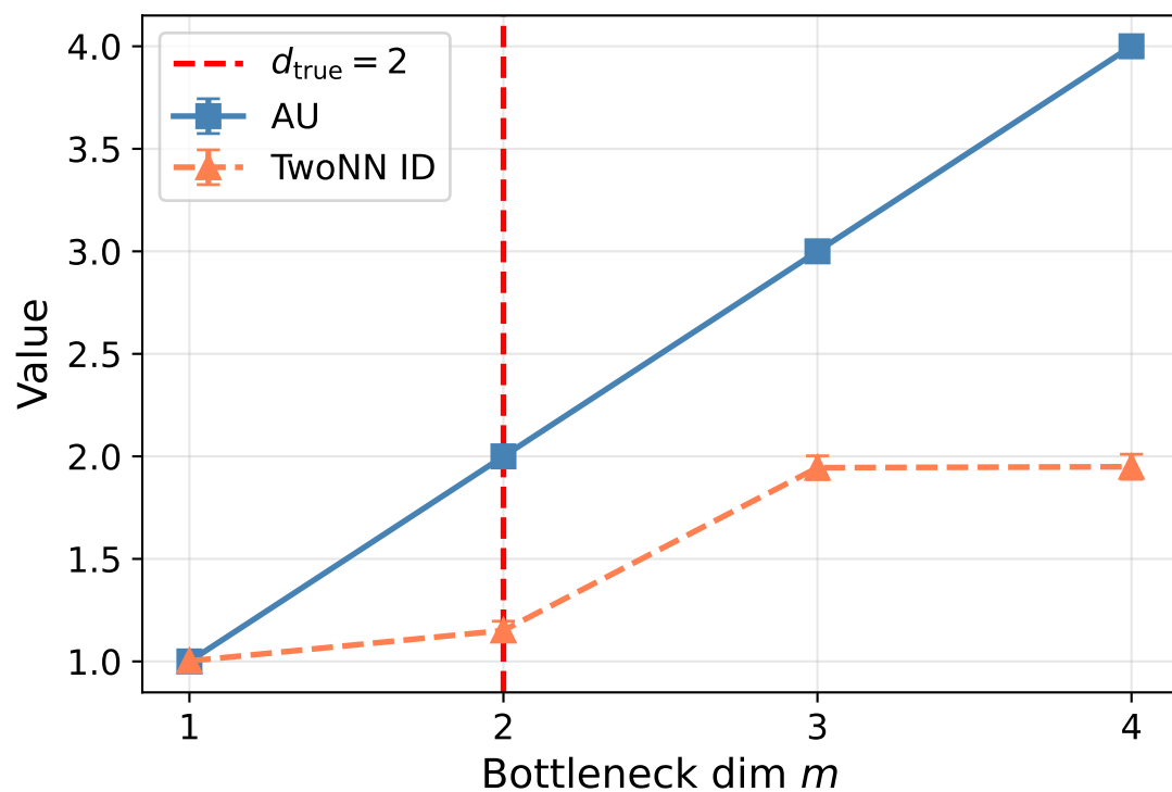
Swiss Roll: AU & ID vs m
