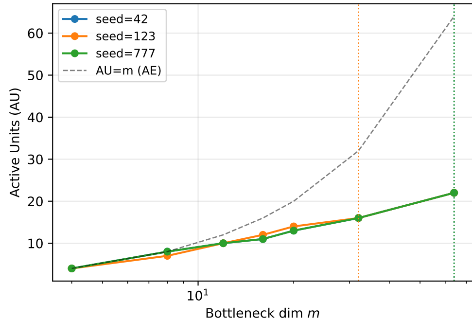
VAE AU vs m (3 seeds)
