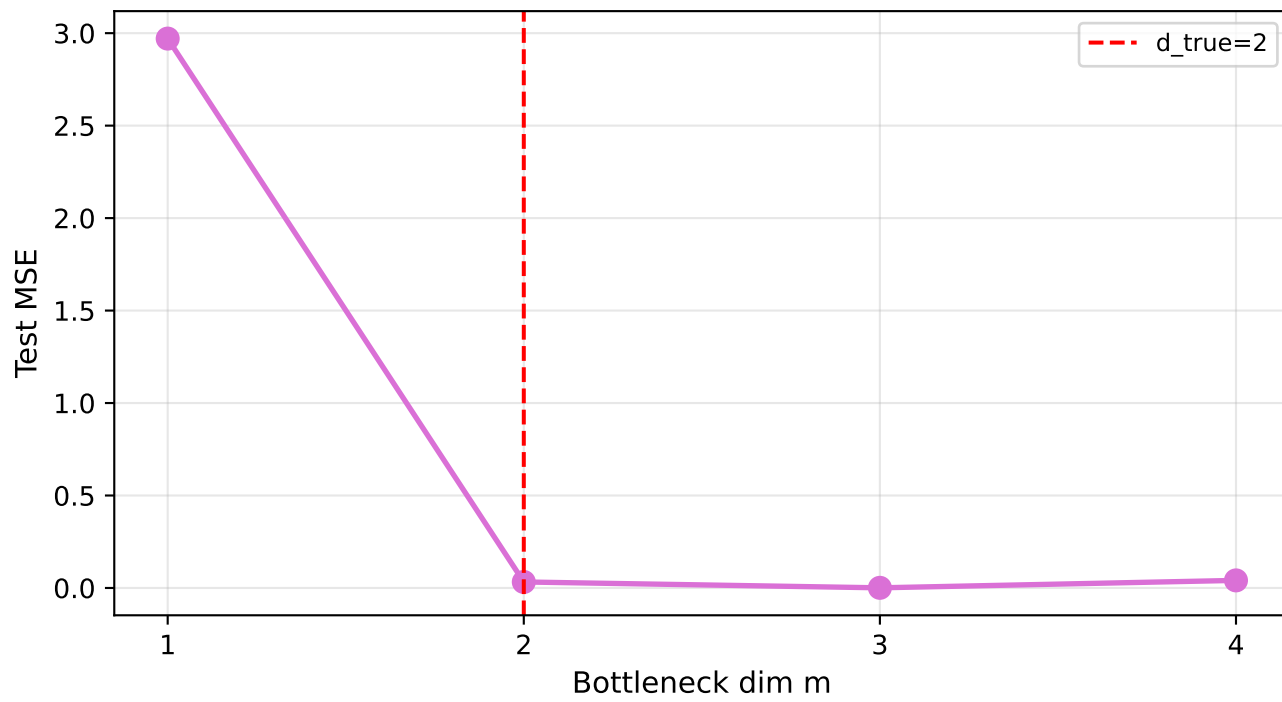
SwissRoll: Test MSE
