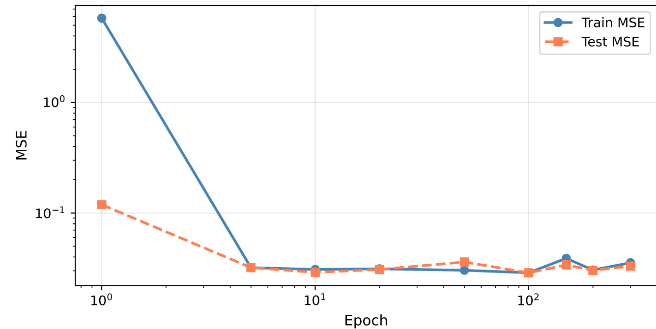
Reconstruction MSE
