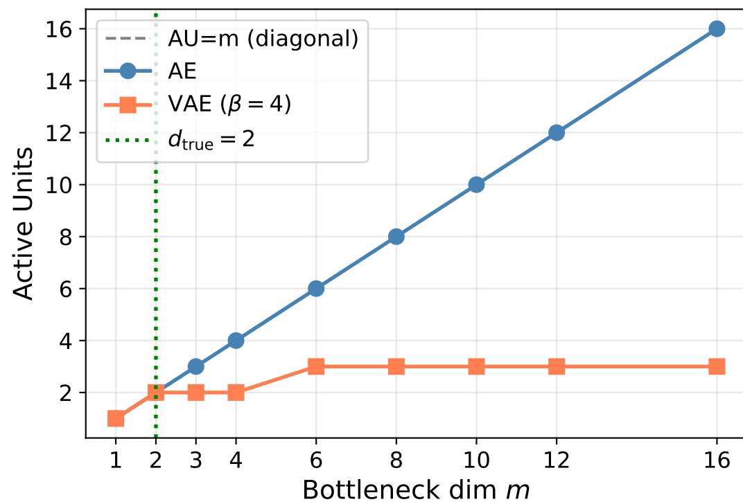
Torus: AU vs m
