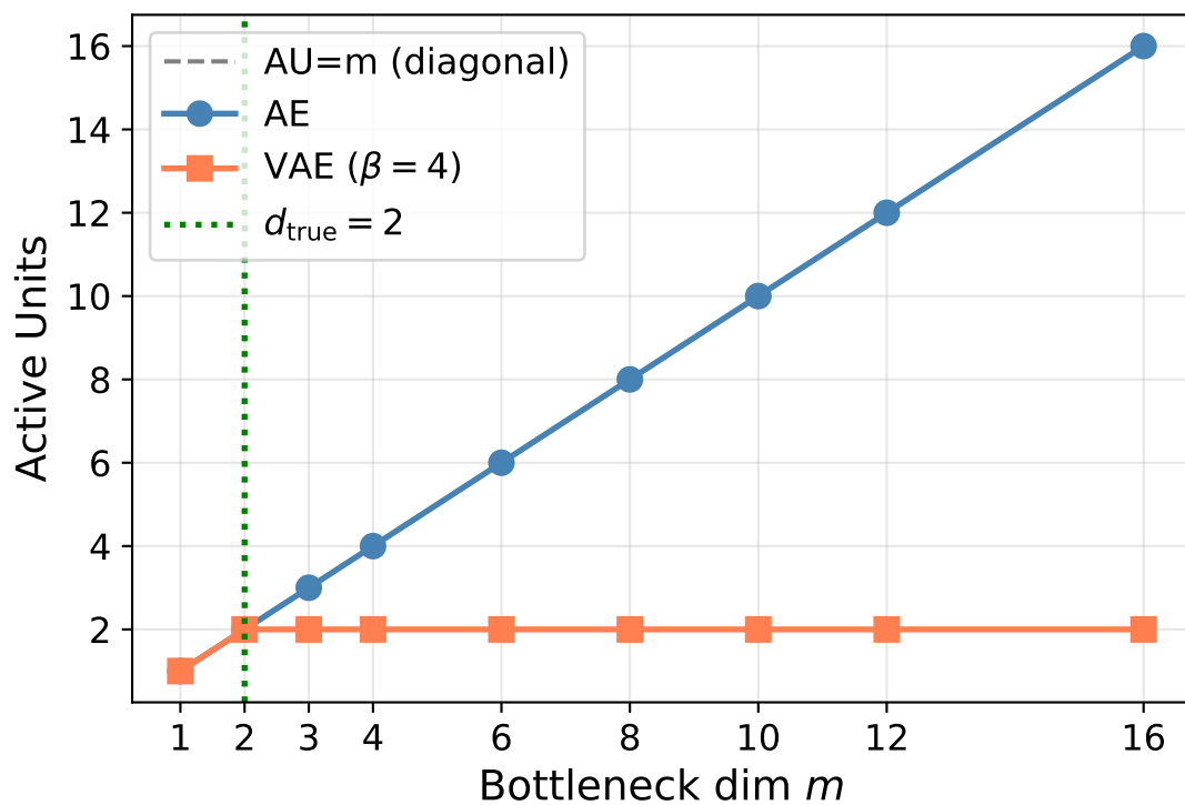
SwissRoll: AU vs m
