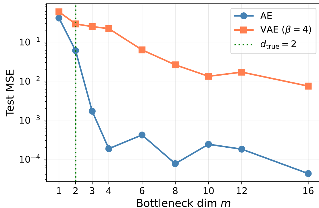
Torus: MSE vs m
