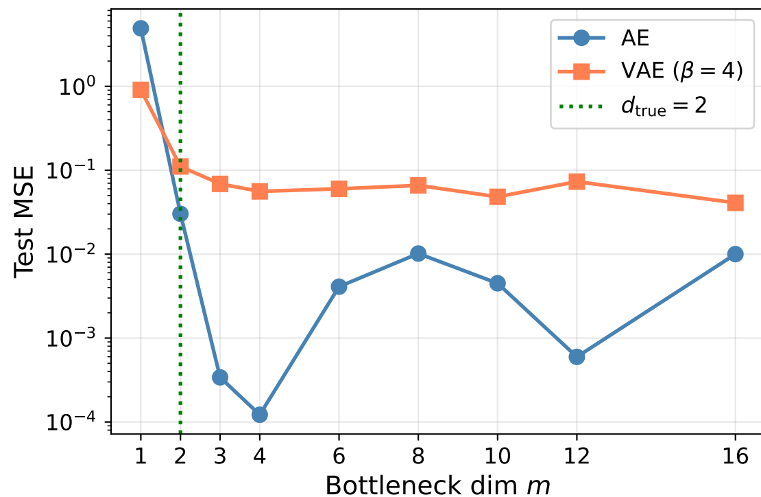
SwissRoll: MSE vs m
