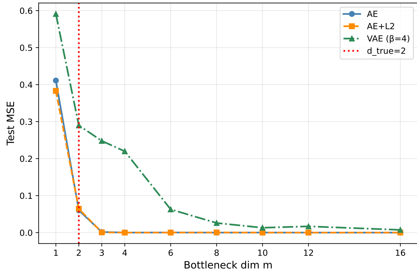
Torus: MSE vs m
