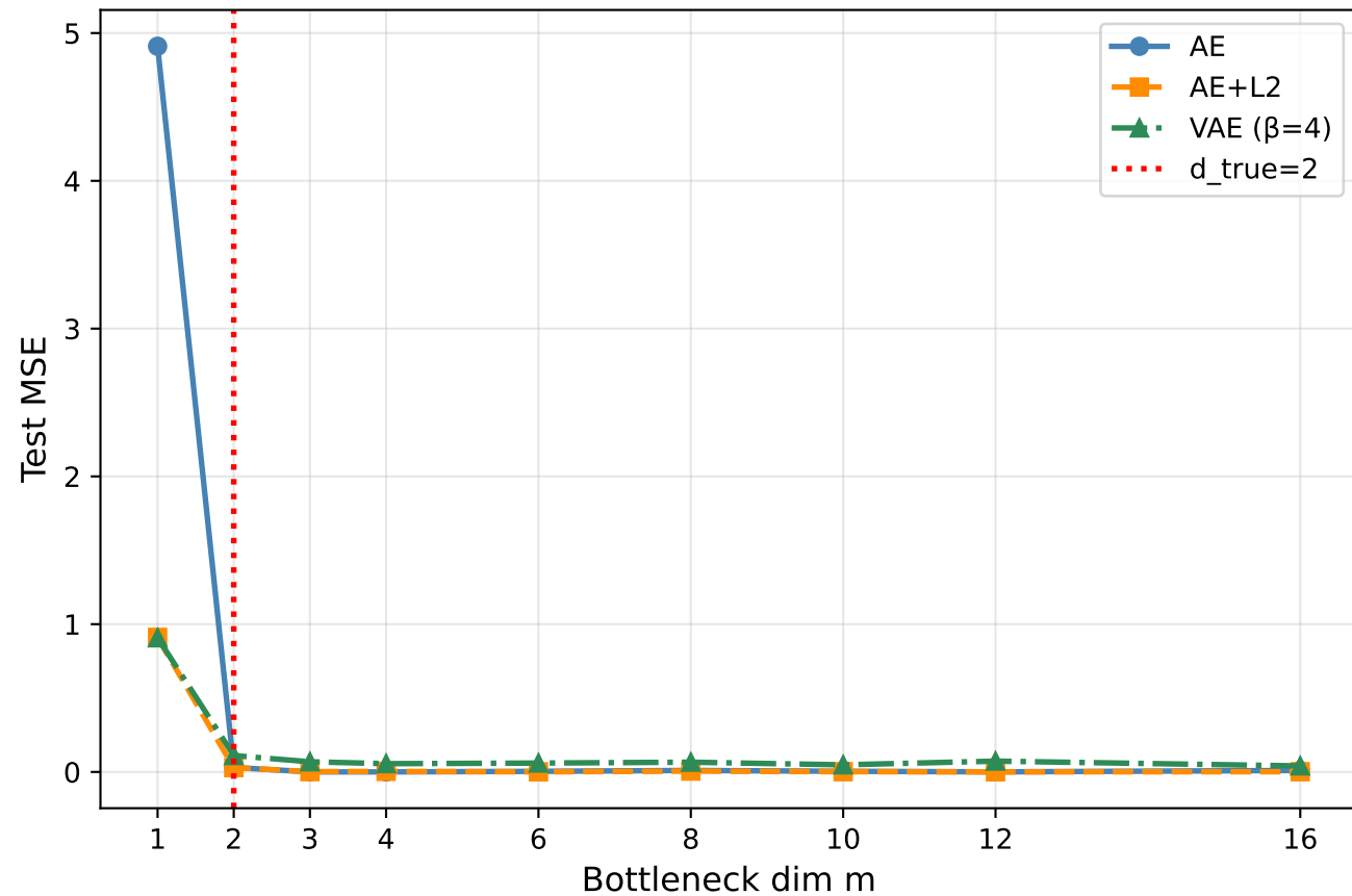
SwissRoll: MSE vs m
