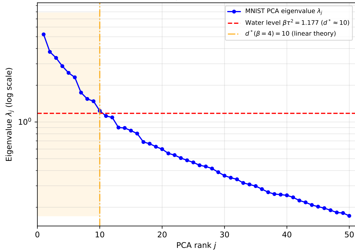
MNIST PCA spectrum: \lambda_j vs. j
