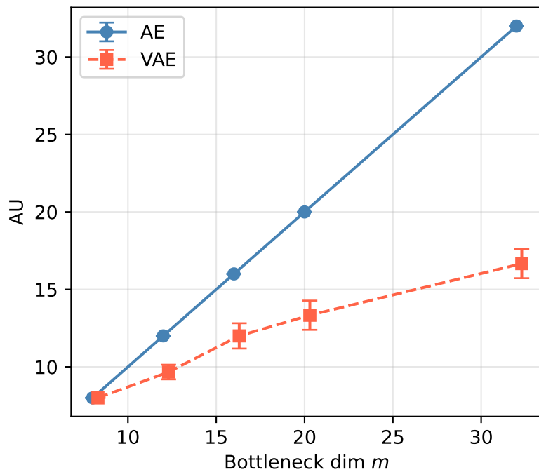
MNIST AU (mean \pm std, 3 seeds)
