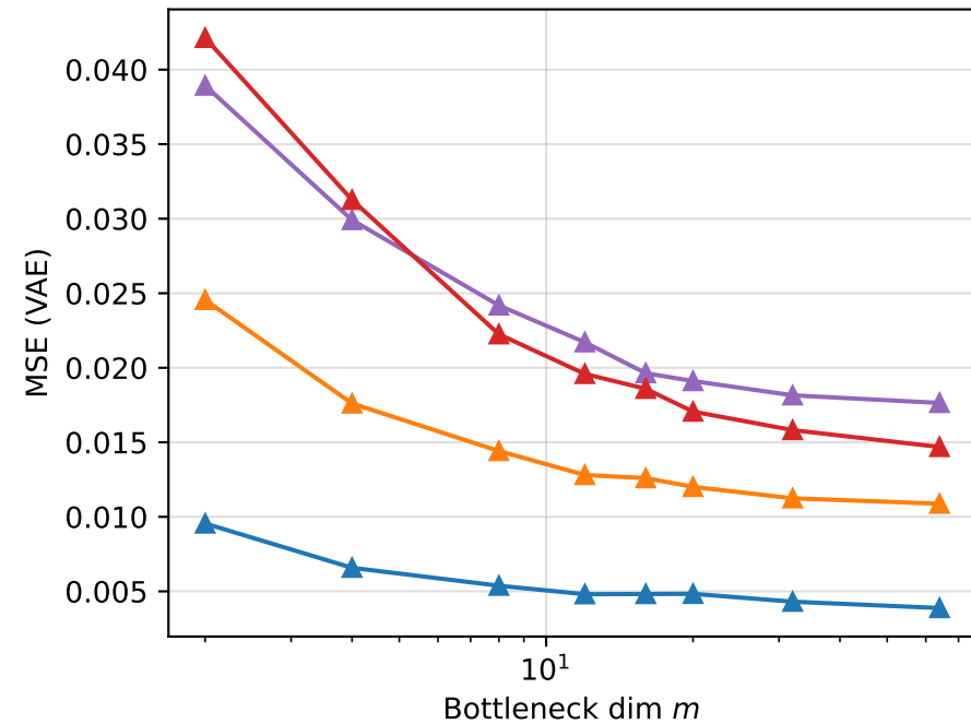
MSE vs m
