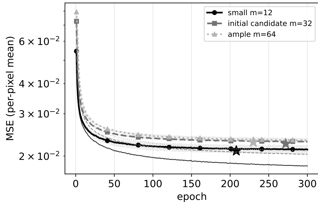
MNIST: reconstruction MSE
