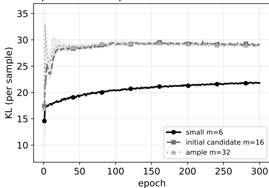
dSprites: KL term
