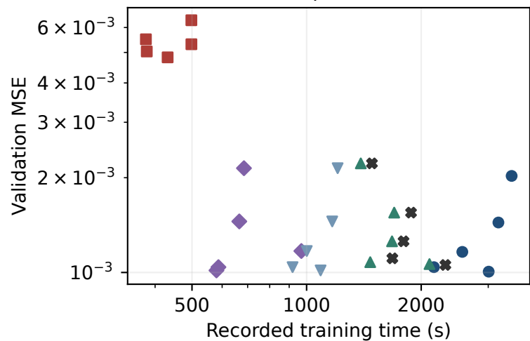
dSprites
