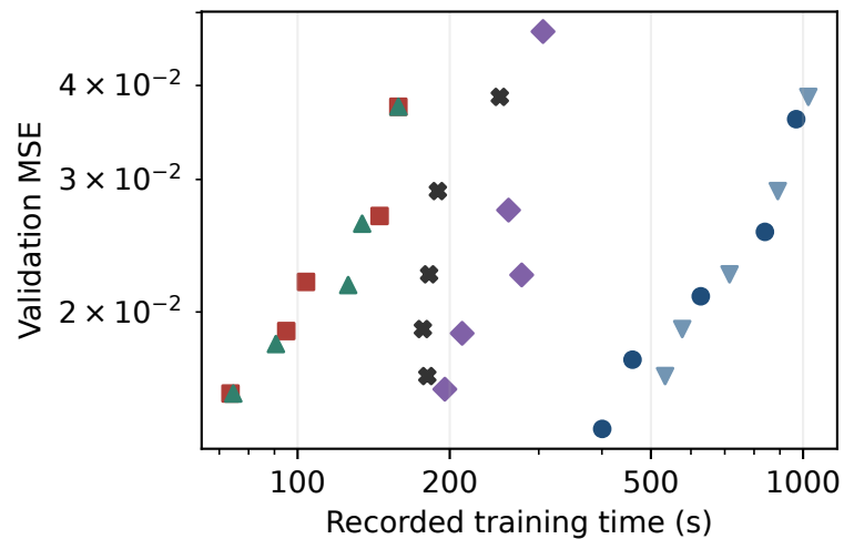
dSprites
