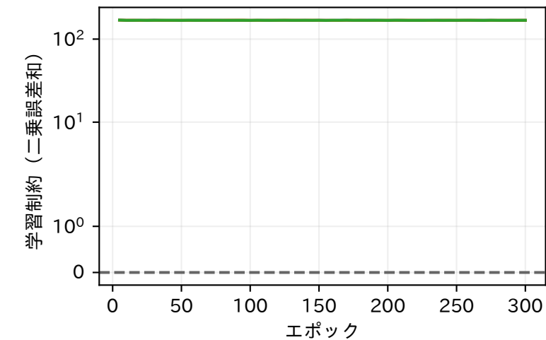
dSprites
