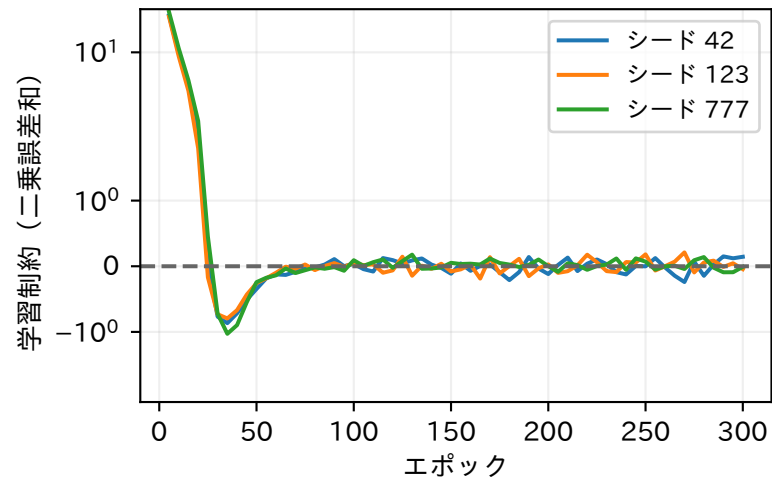
dSprites
