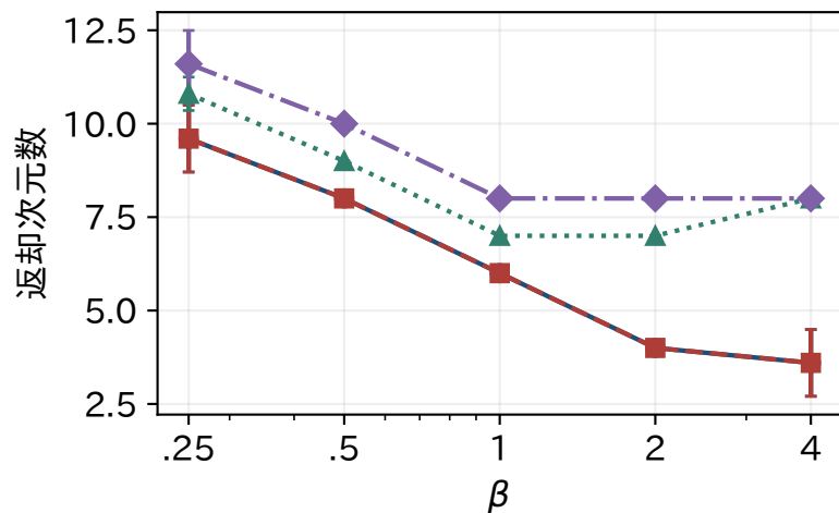
dSprites
