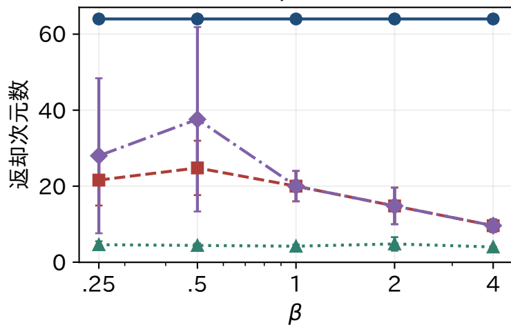
dSprites
