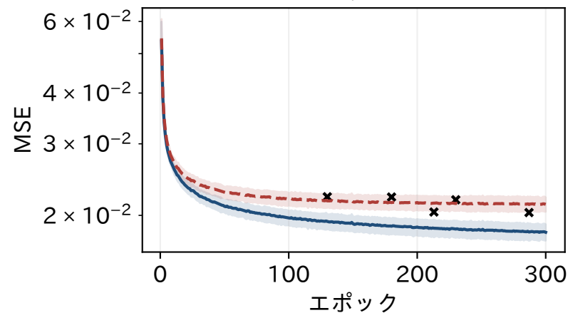
MNIST, m=32
