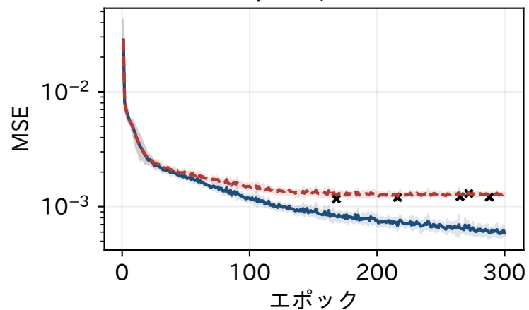
dSprites, m=32
