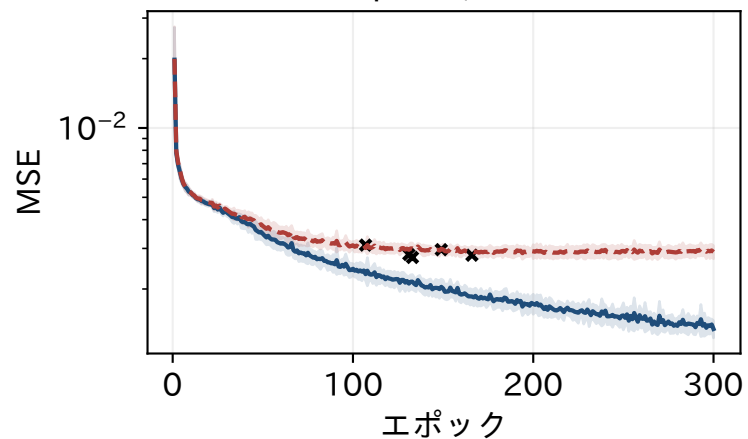
dSprites, m=16
