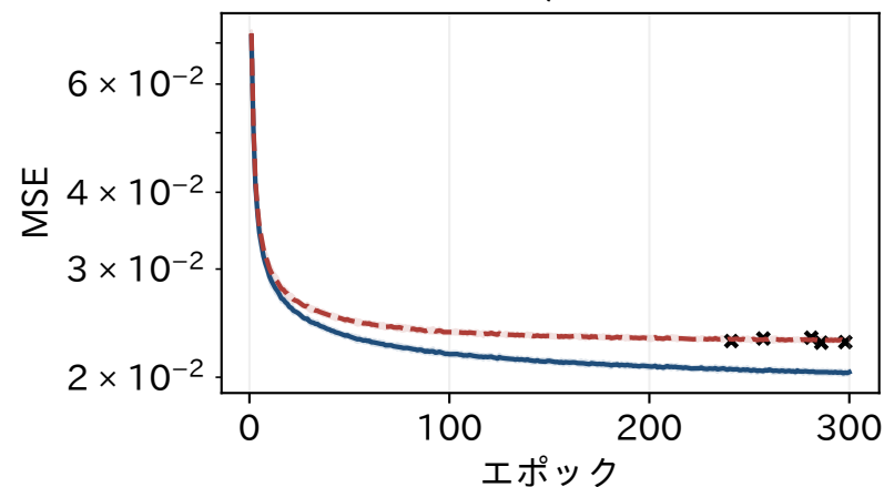
MNIST, m=64
