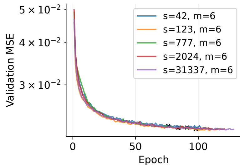
dSprites
