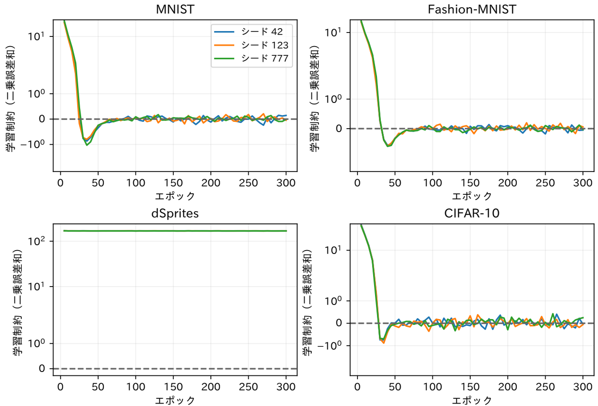
図 A3: 新しい ARM 各シードの確率的学習制約の移動平均。5 epochs ごとに記録した。ゼロが制約境界で, 負値は制約充足を表す。大きな正の違反量と負値を表示するため, 縦軸は対称対数尺度とする。これらの推移は, 決定的な検証目標の達成とは異なる。
