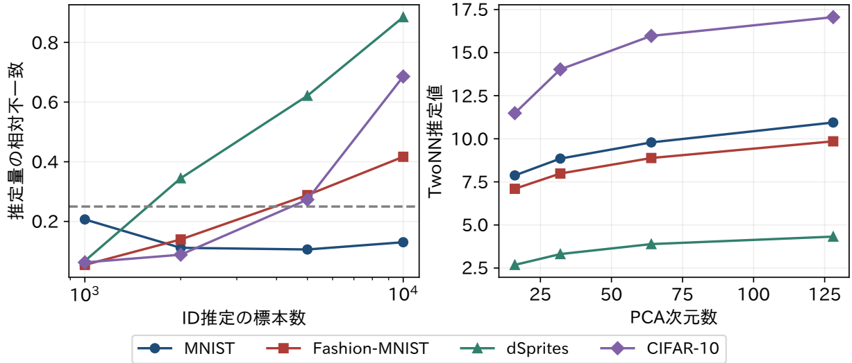
図 1: 左: 推定標本数を変えた生入力での |d_{\text{TwoNN}} - d_{\text{MLE}}|/d_{\text{TwoNN}} 。破線は 0.25。右: PCA 前処理後の TwoNN。PCA 次元, 標本数, 表現は別の介入であり, AE 結果は表 12 に示す。
