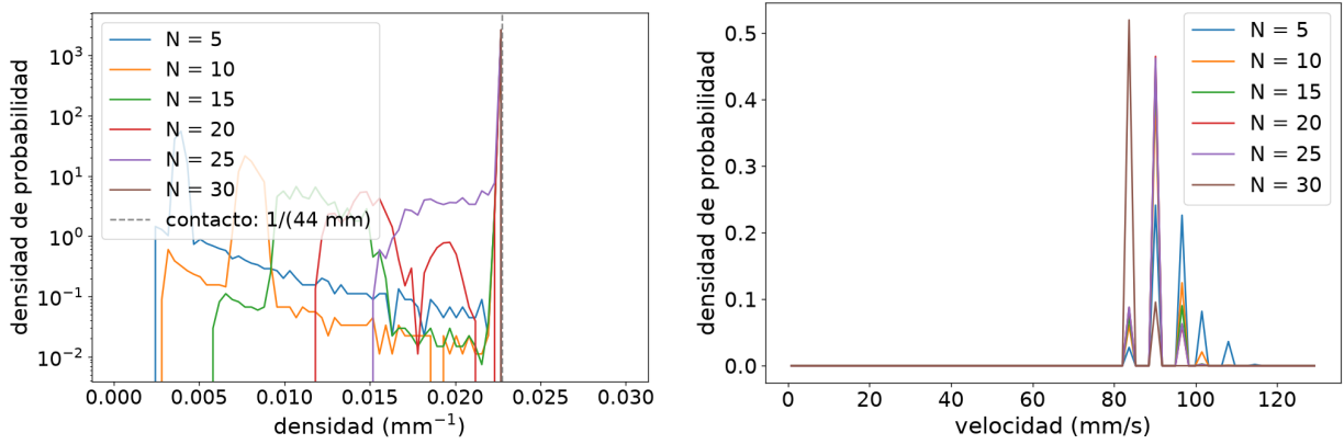
Figura 4: Distribuciones (PDF) de densidad individual (izquierda; pico en 1/(44 \text{ mm}) ) y de velocidad microscópica (derecha), una curva por N ( N fijo, contacto puro, p = 0,1 ).
