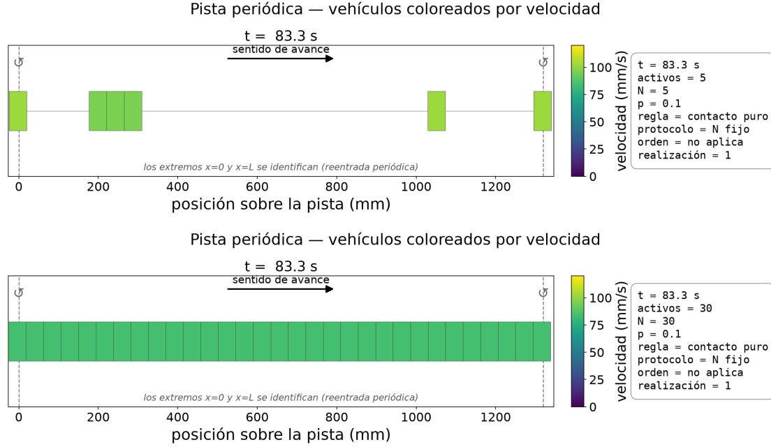
Figura 1: Fotogramas en régimen a baja densidad ( N = 5 , arriba) y a saturación ( N = 30 , abajo), contacto puro, p = 0,1 . Color según velocidad. Animaciones disponibles en el repositorio del grupo.
