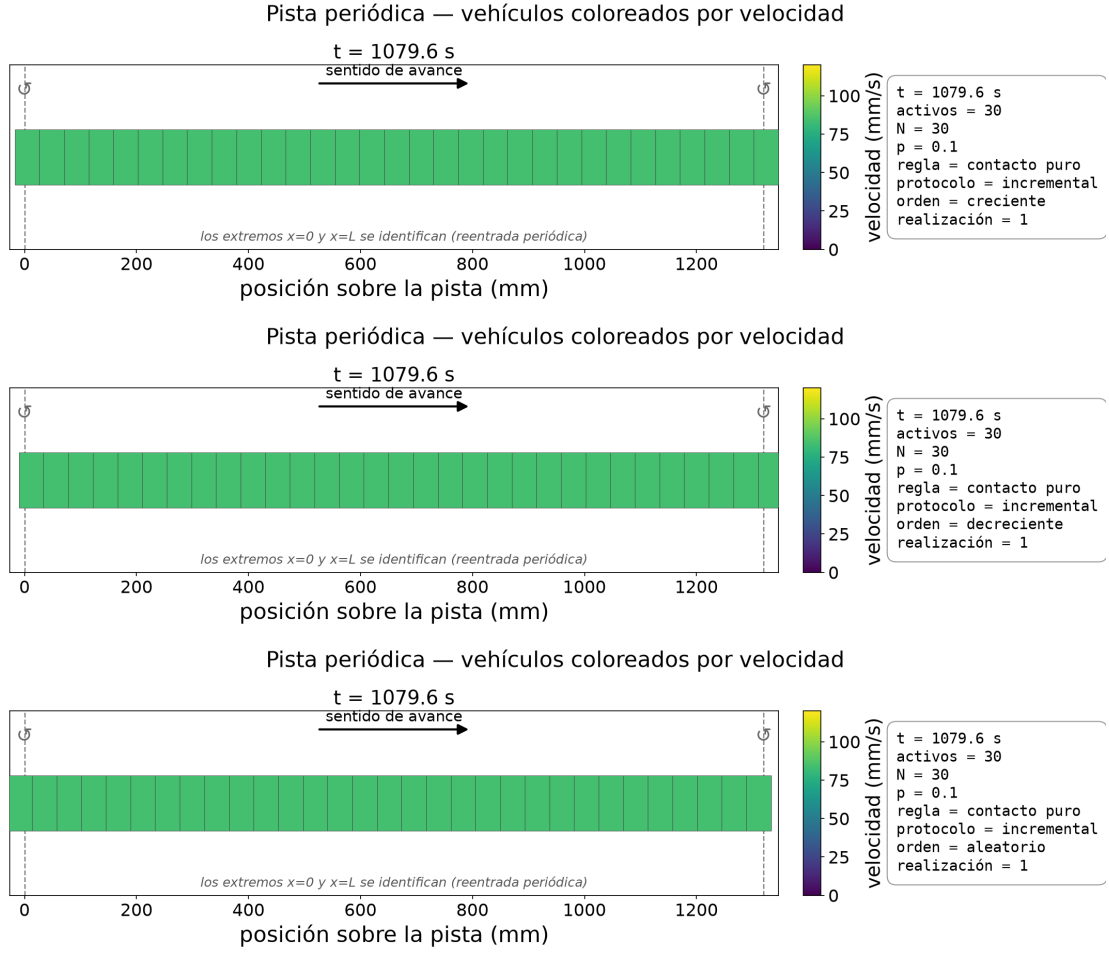
Figura 6: Fotogramas del protocolo incremental para los órdenes creciente (arriba), decreciente (medio) y aleatorio (abajo) (contacto puro, p = 0,1 ). Animaciones disponibles en el repositorio del grupo.
