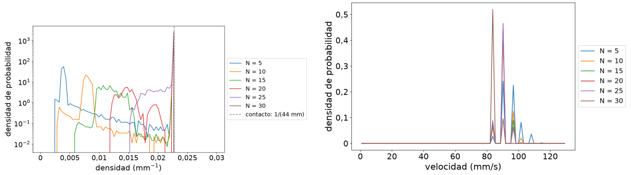
Figura 4: Distribuciones de densidad individual (izquierda; pico en 1/(44 \text{ mm}) ) y de velocidad microscópica (derecha), una curva por N ( N fijo, contacto puro, p = 0,1 ).
