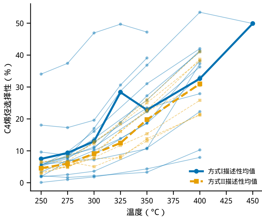
各组合温度响应及装料方式描述性均值
