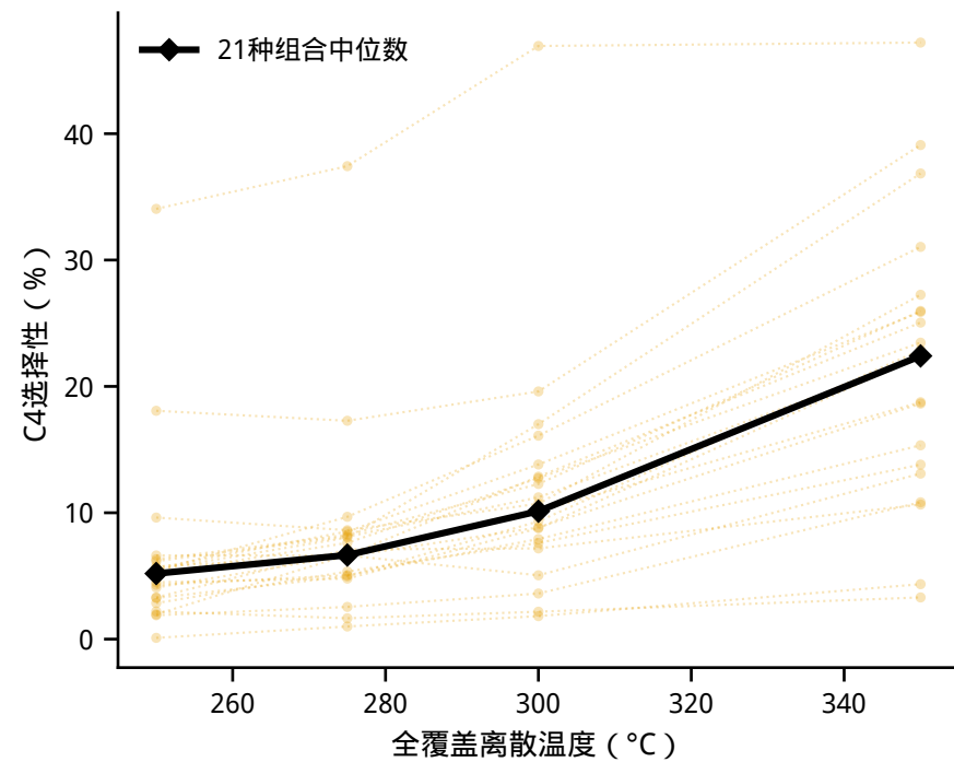
四个全覆盖温度条件下的组合内响应比较（连线仅辅助观察）
