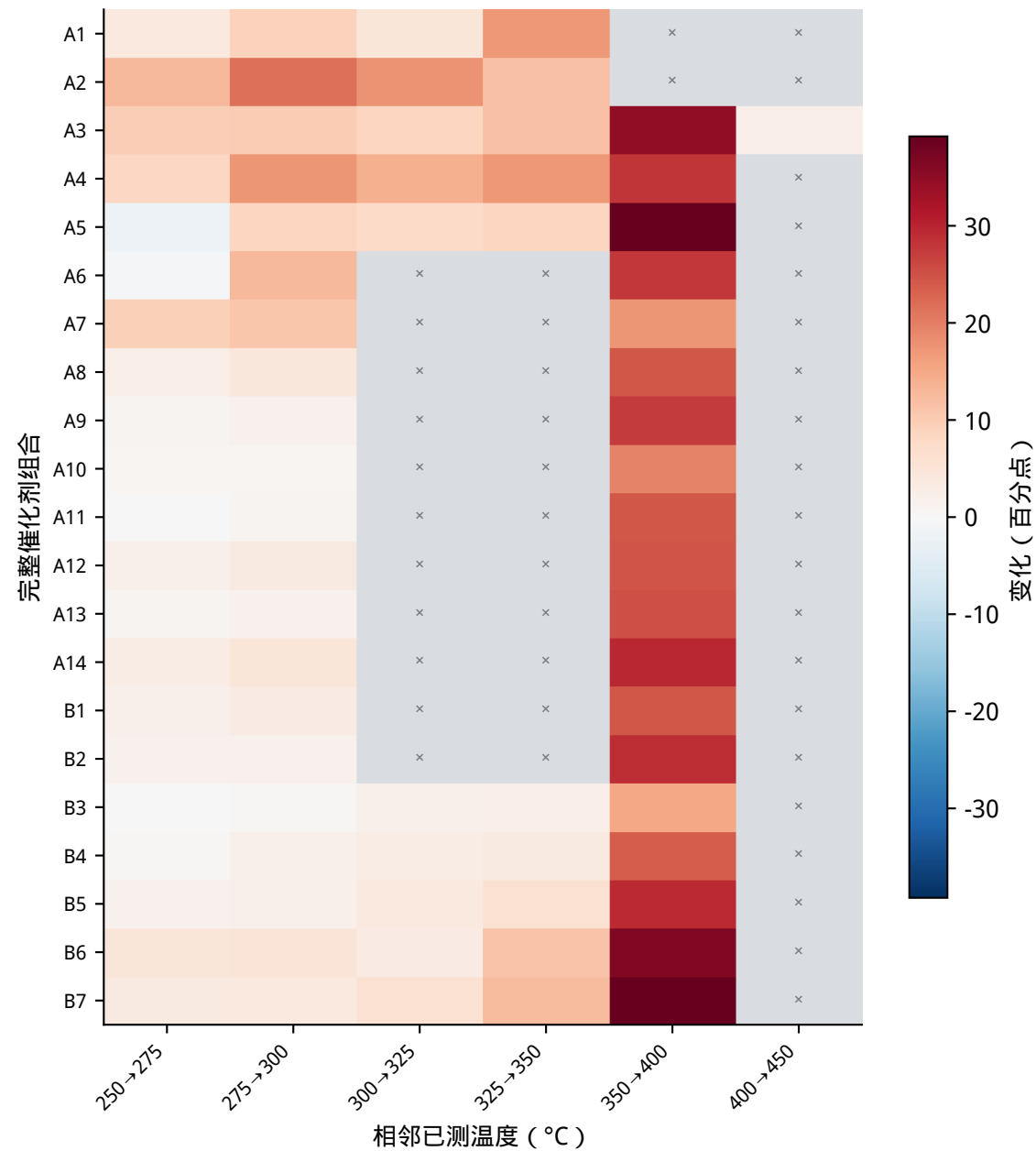
乙醇转化率
