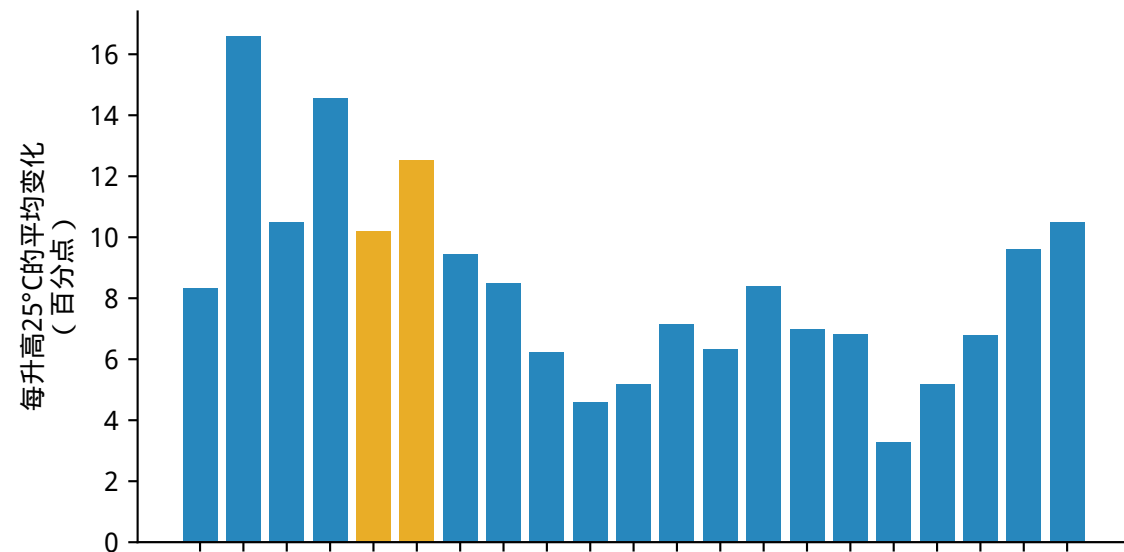
乙醇转化率
