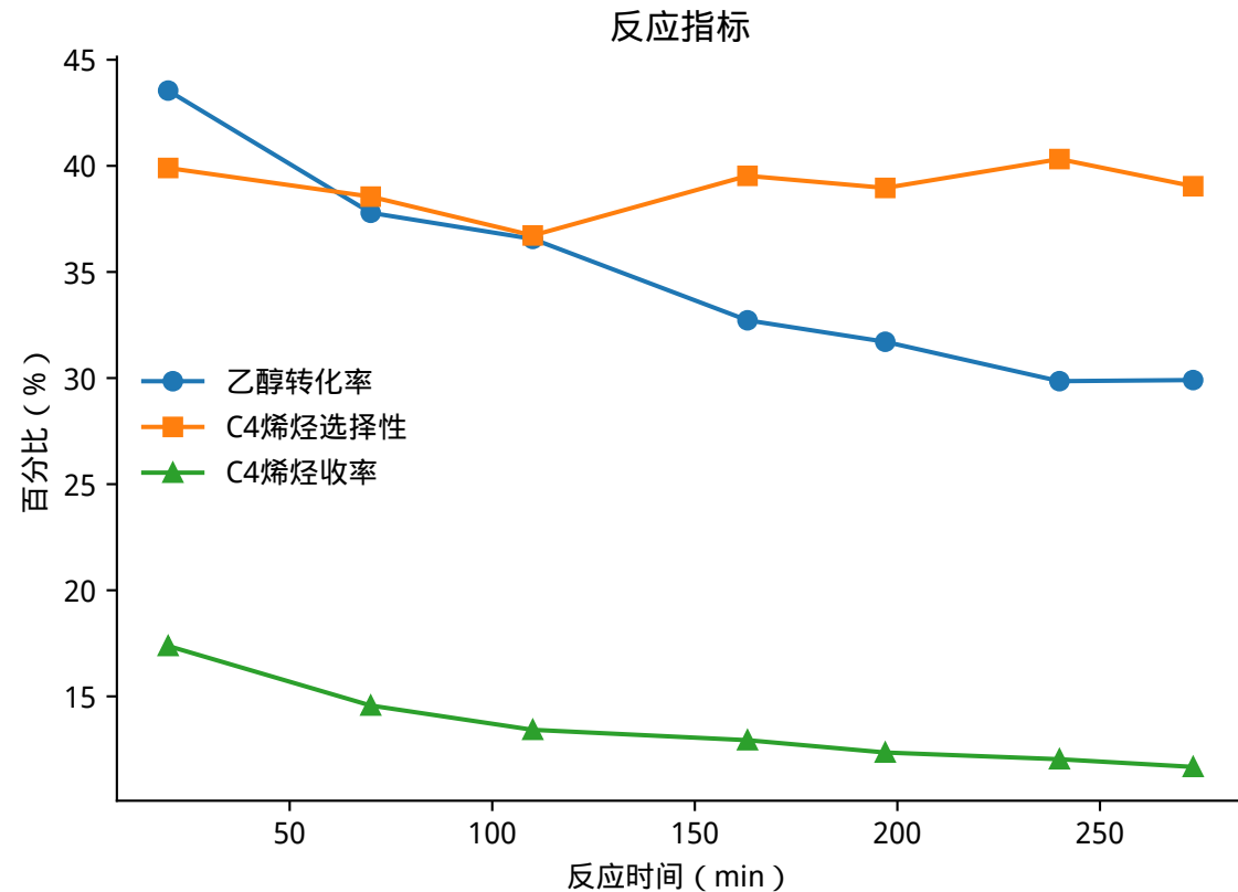
350°C下各反应指标及产物选择性随时间的变化
