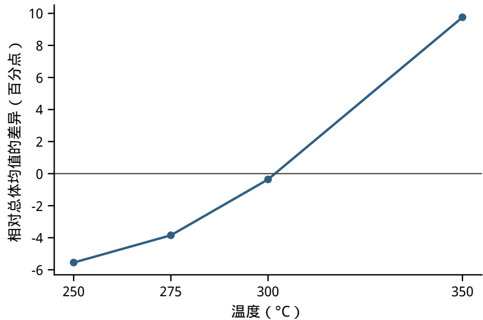
C4 烯烃选择性
