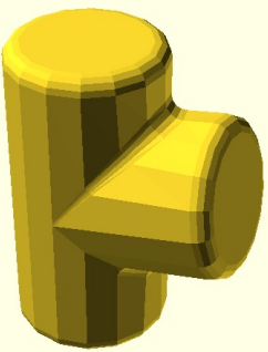
S1-T04 tee_oblique (fn=16) VALID warnings=0
