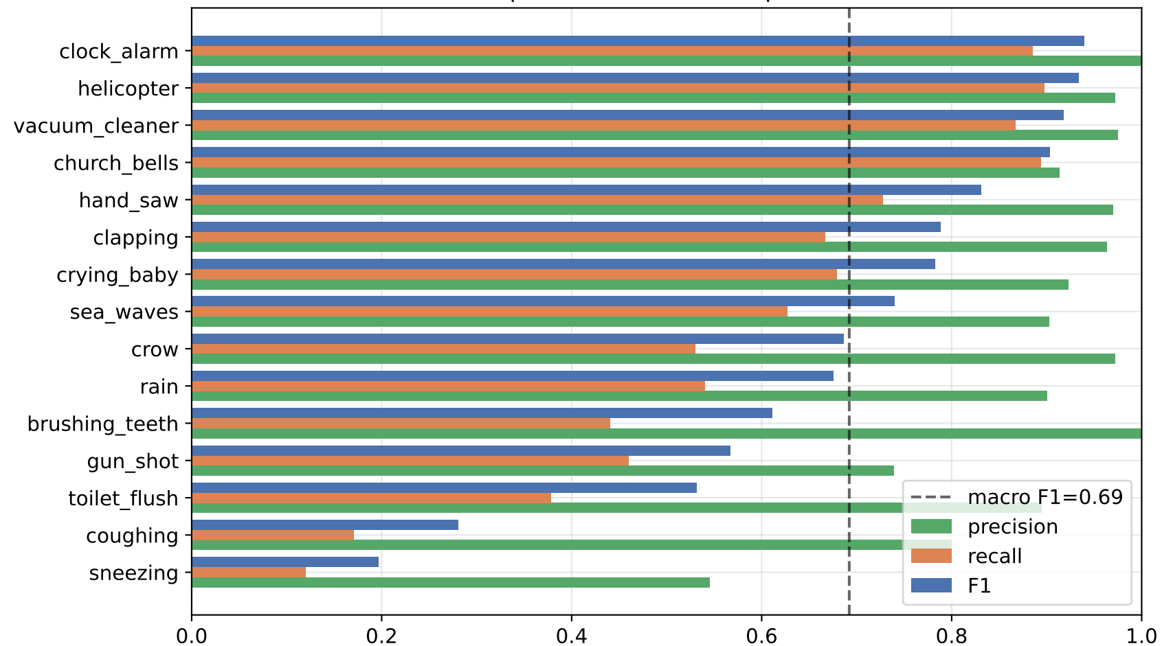
Detection precision / recall / F1 per class - v3.0
