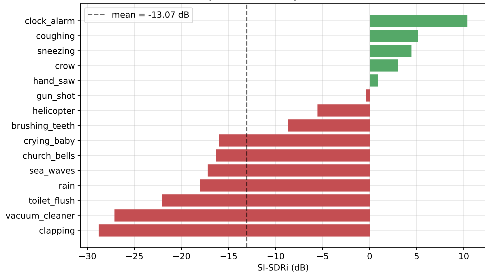
Separation SI-SDRi per class - v3.0
