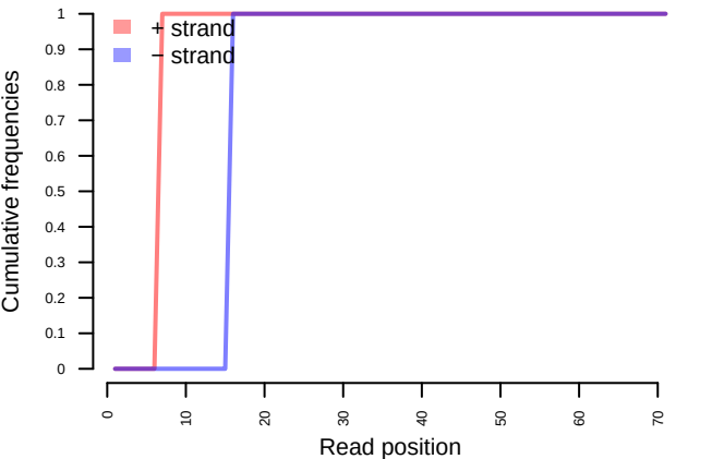
C>T
