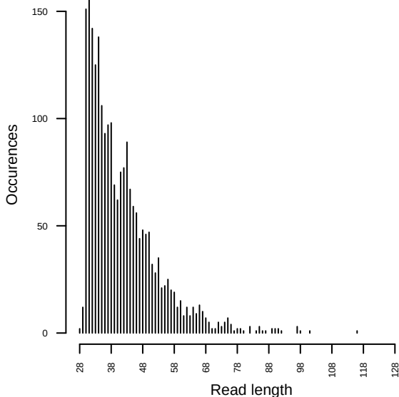
C>T
