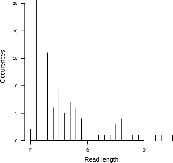
C>T
