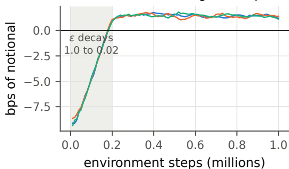
(d) Double DQN: training reward per window
