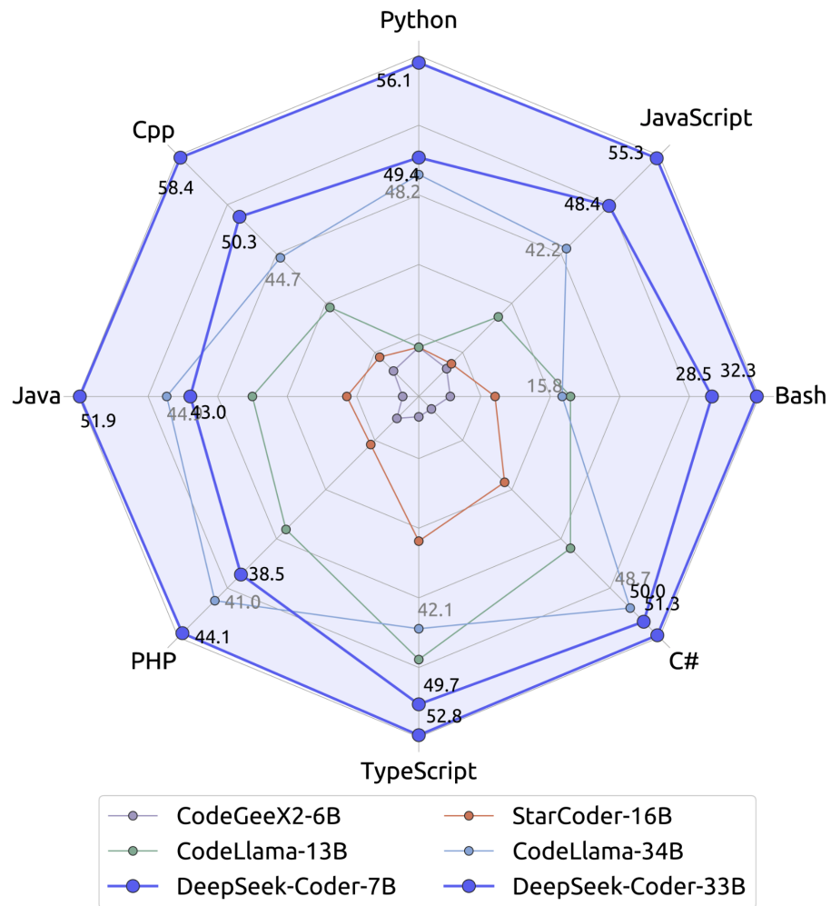
Figura 6.1: Grafico de comparación del rendimiento con respecto otros modelos open source basados en código [4]
