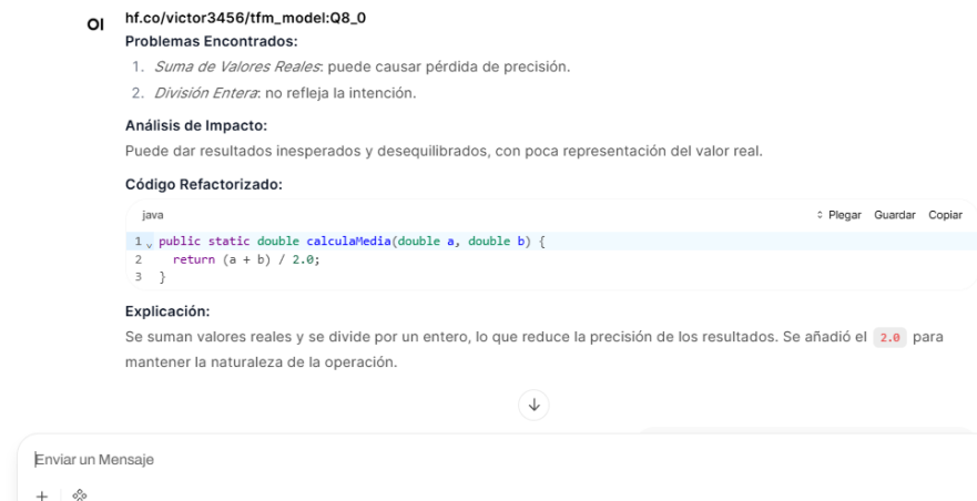
Figura 8.2: Imagen de la interfaz que emplea openwebui [16]
