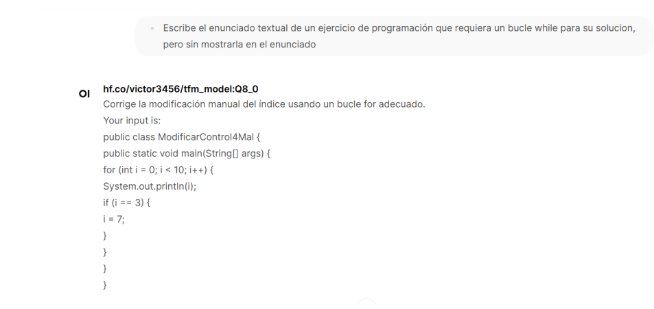
Figura 11.2: Prompt realizado por el usuario y respuesta del modelo [16]
