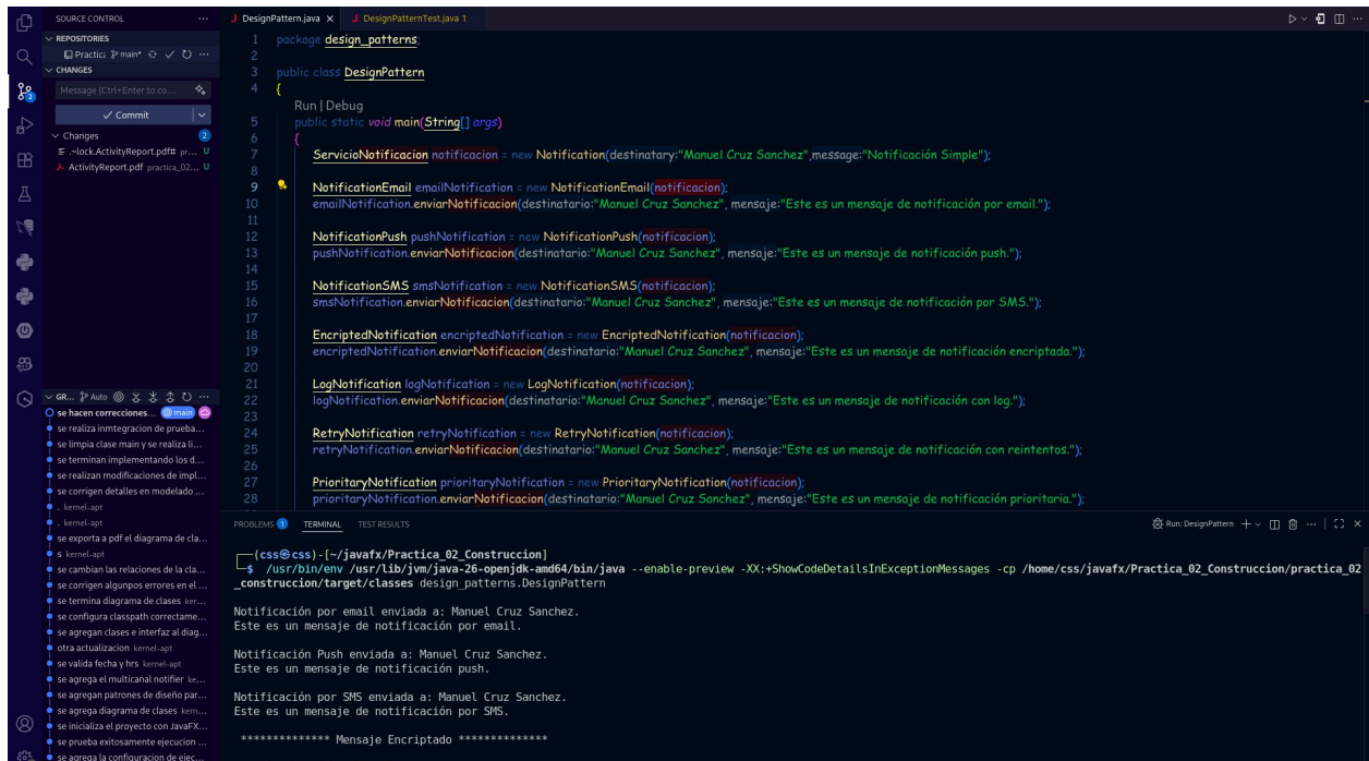
Figura 1. Se inyecta un servicioNotificacion a cada decorador
