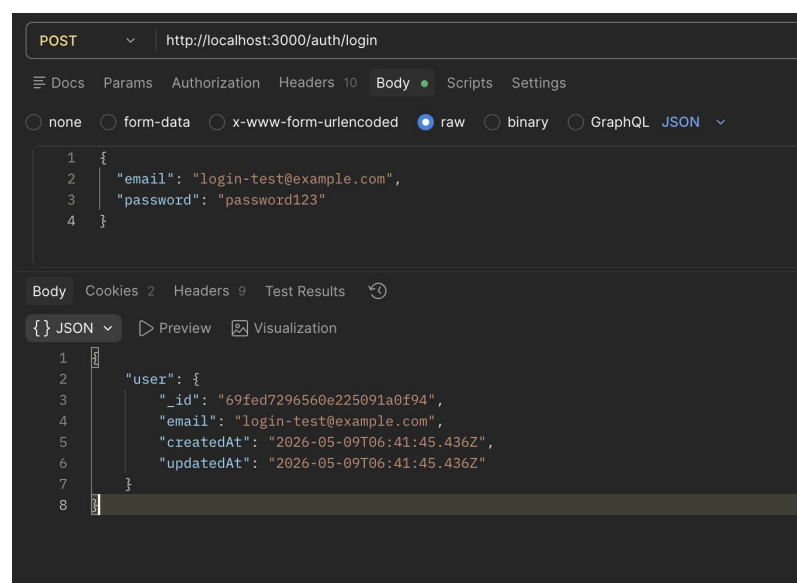
Рис 6. Вхід користувача в систему
