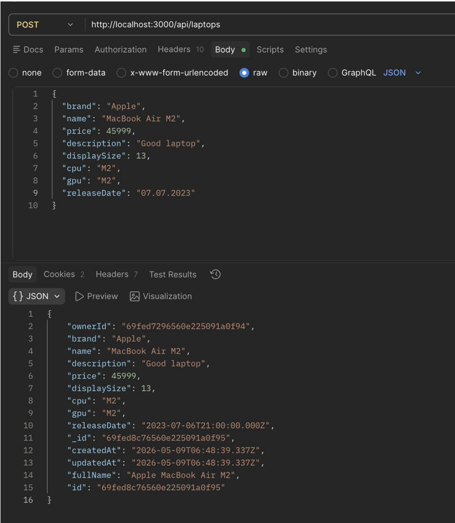
Рис 14. Створення ноутбуку після авторизації
