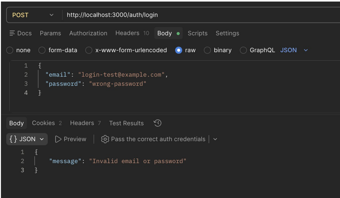
Рис 8. Введення неправильного паролю
