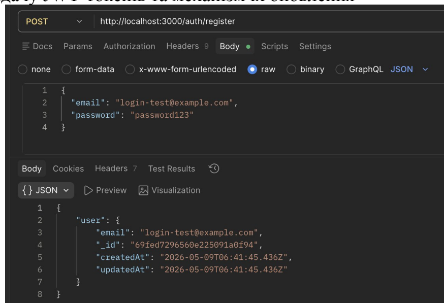
Рис 5. Створення користувача через postman
