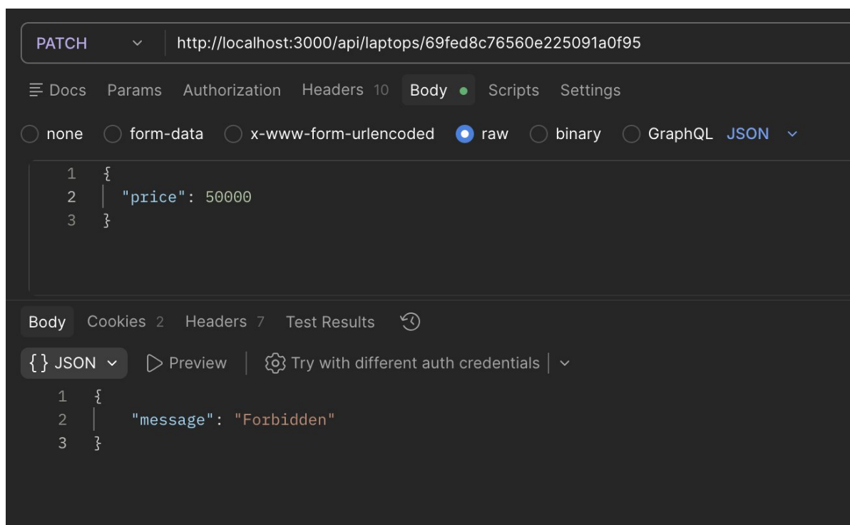
Рис 18. Спроба змінити чужий ноутбук
