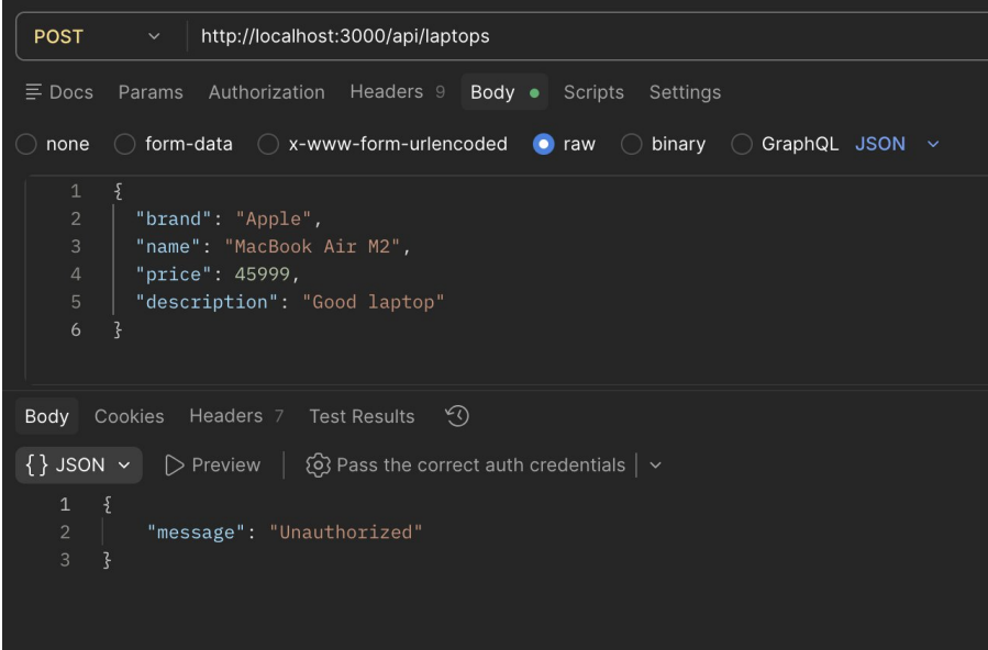
Рис 13. Спроба створити ноутбук без авторизації
