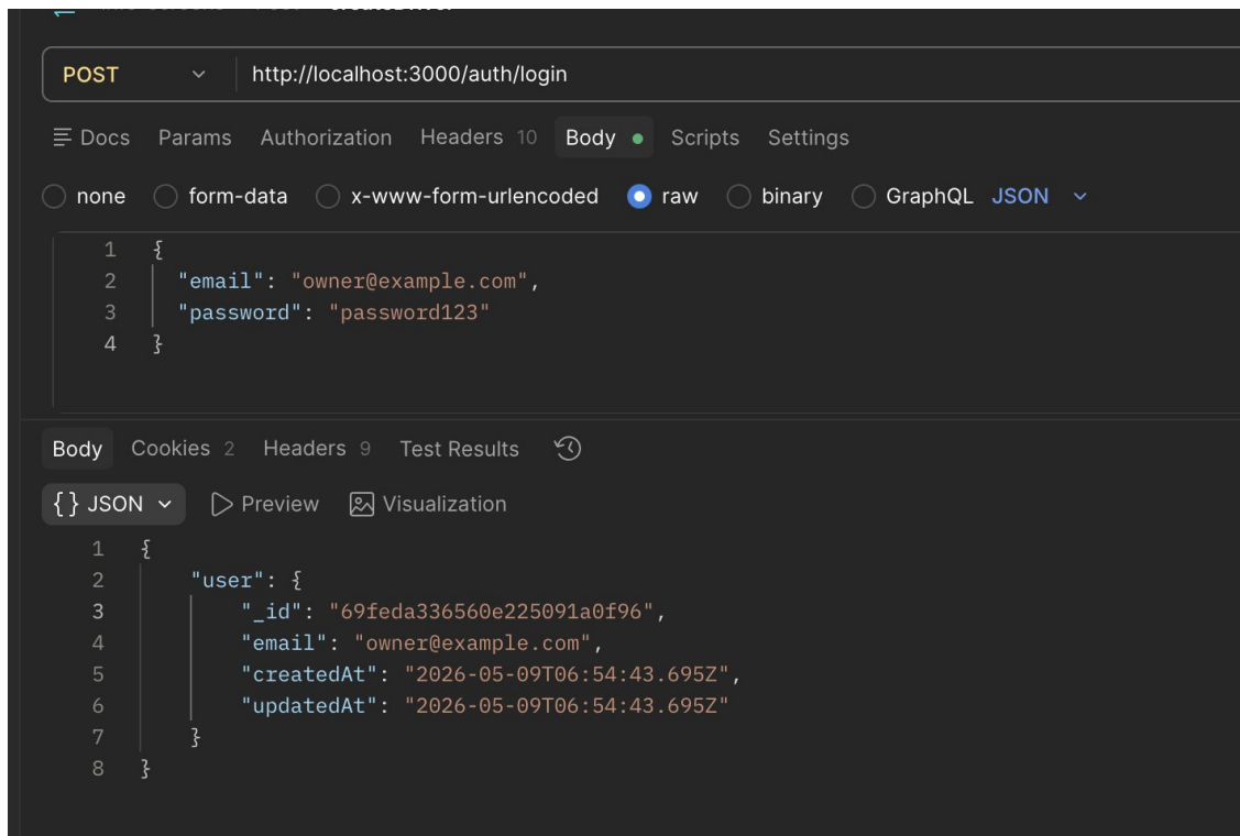
Рис 17. Вхід в систему під новим користувачем
