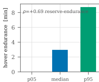
eVTOL: 3.1C hover
