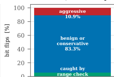
orbiter: 40,000 SEU flips
