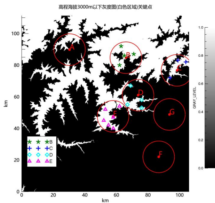
图 4-11 高程海拔 3000 米以下灰度图关键点选择
