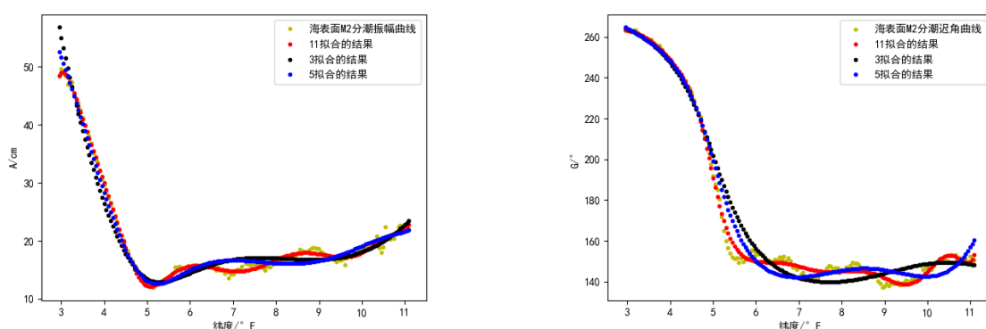
图 5-28 25 号轨道分潮 M2 拟合振幅、迟角结果
