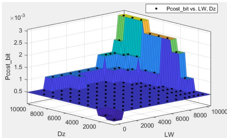
图 10 导频开销与色散、线宽关系图
