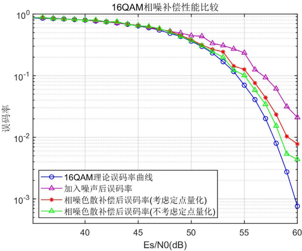
图 11 16QAM 相噪补偿性能比较
