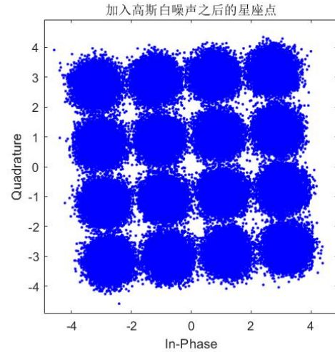
d. 加入高斯白噪声后的星座图
