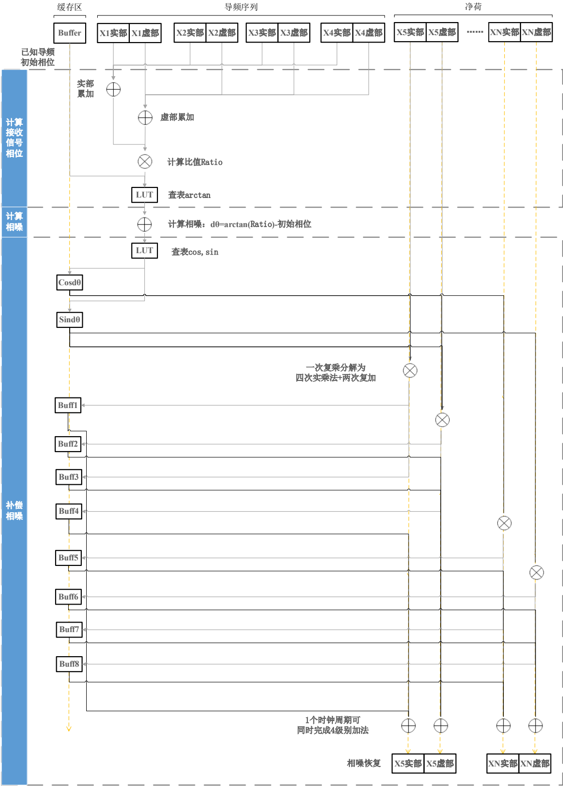
图 7 运算时序图
