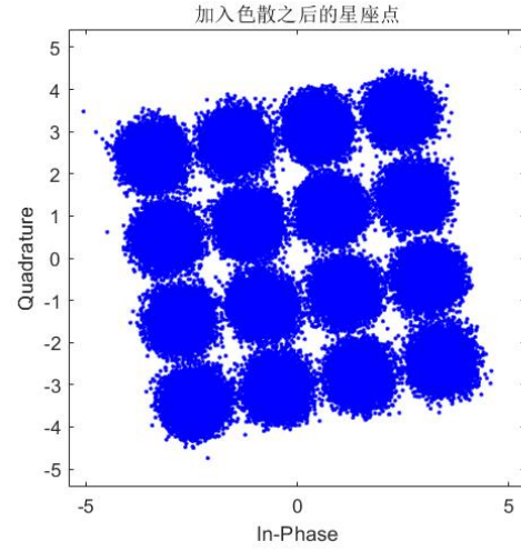
b. 加入色散后的星座图
