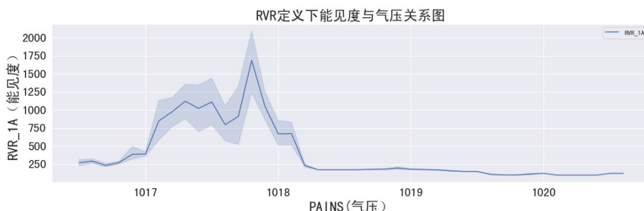
图 10 RVR 定义下能见度与气压关系
