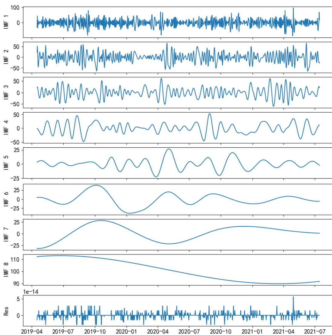
图 15 CEEMDAN 分解结果
