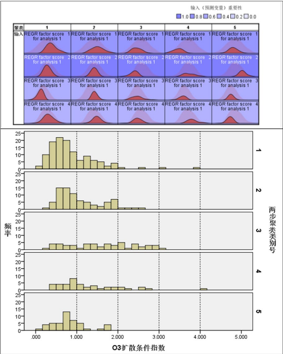
图 7 气象主成分分布特征（上）及各类气象下 O 3 污染扩散条件参数直方图（下）
