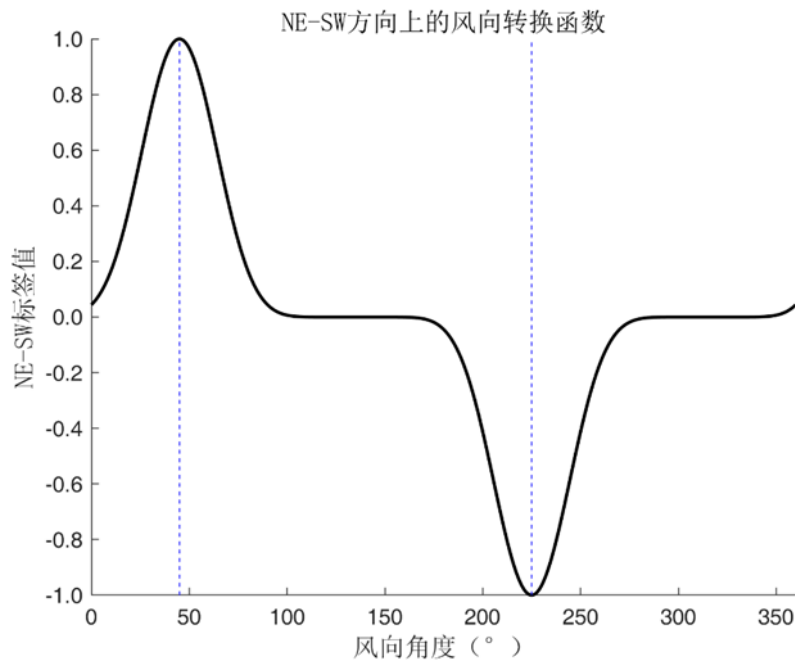
图 2 NE-SW 方向上的风向转换函数
