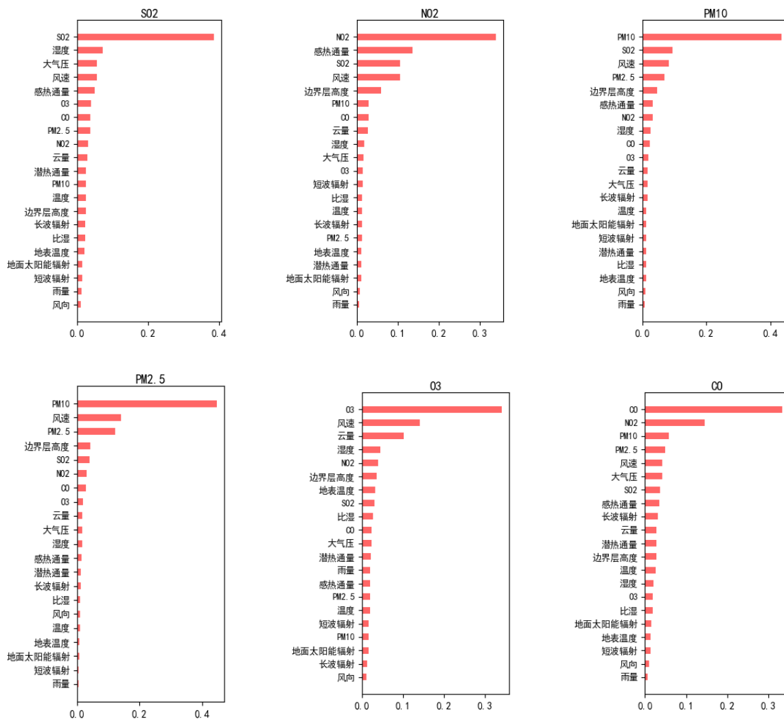
图 9 监测点 A 特征重要度排序情况
