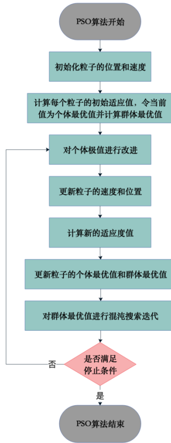
图 44 粒子群优化算法流程图
