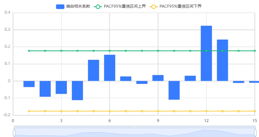
图 60 蒸发量预测模型 PACF 验证图
