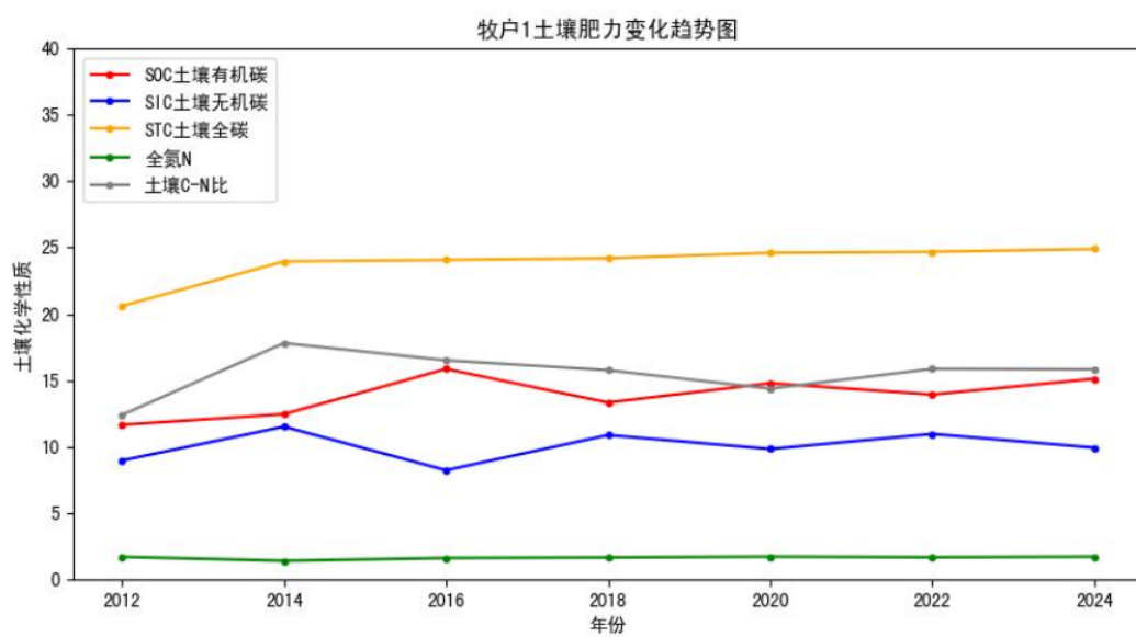
图 53 牧户一土壤肥力变化趋势观测图
