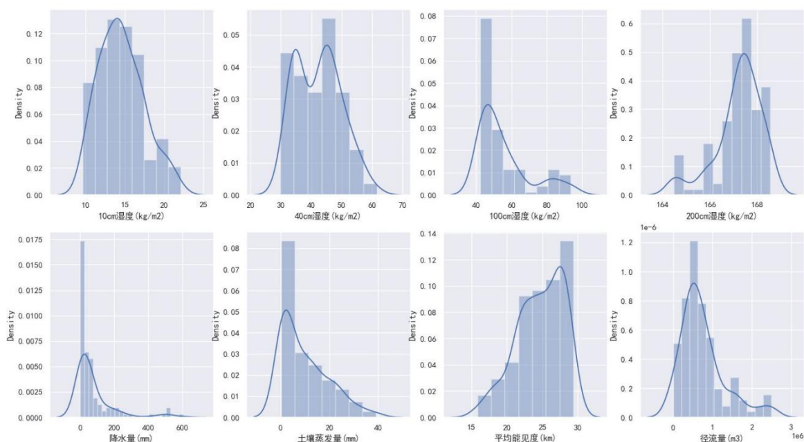
图 18 不同湿度和四个特征的分布范围图
