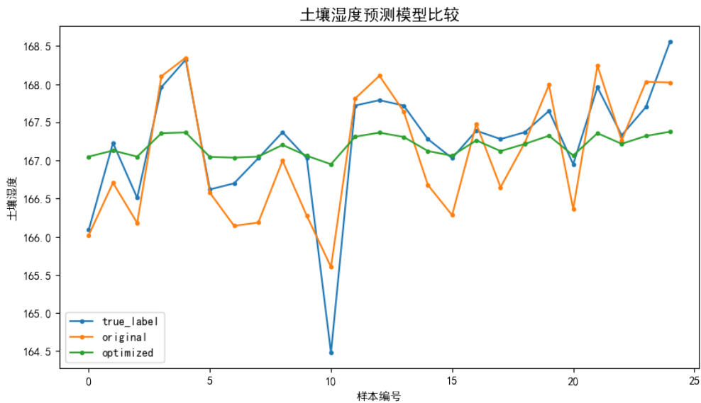
图 6 土壤湿度预测对比
