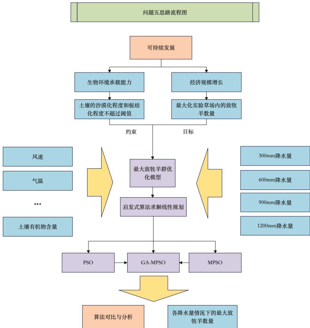
图 43 问题五的思路流程图
