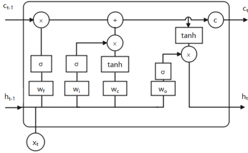
图 21 LSTM 结构图
