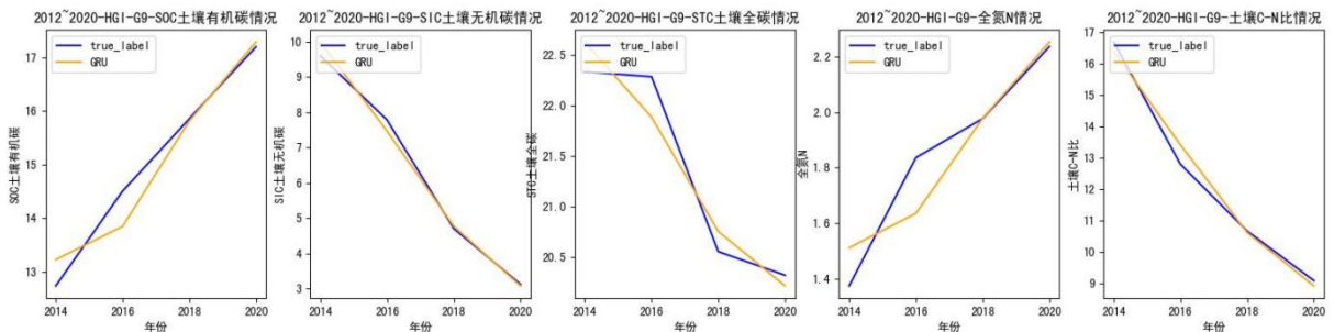
图 37 HGI-G9 的五个土壤化学性质特征预测结果比较图
