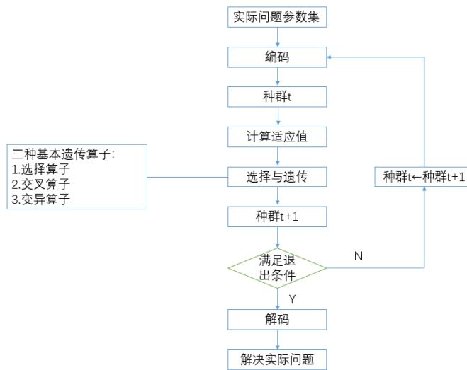
图 5.3 遗传算法流程
