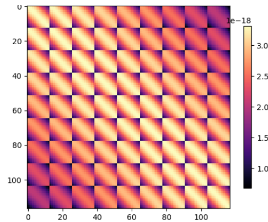
Test2: L^T L + \lambda \text{diag}(L^T L)
