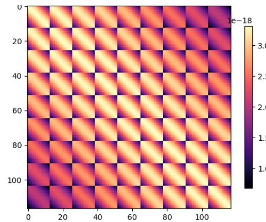
Test2: L^T L + \lambda \text{diag}(L^T L)
